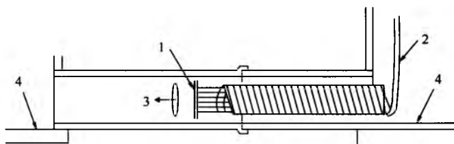
图 24 非贴合螺旋缠绕工艺
